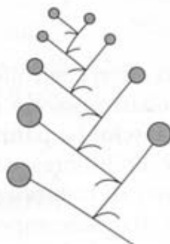
Cima elicoide
