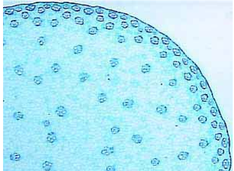
atactostele
