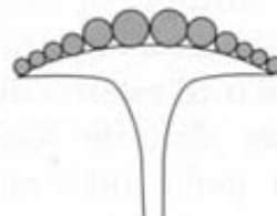
Capolino (= calatide)
