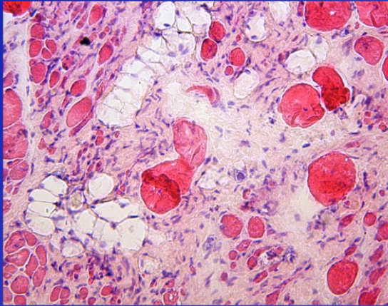
H&E
