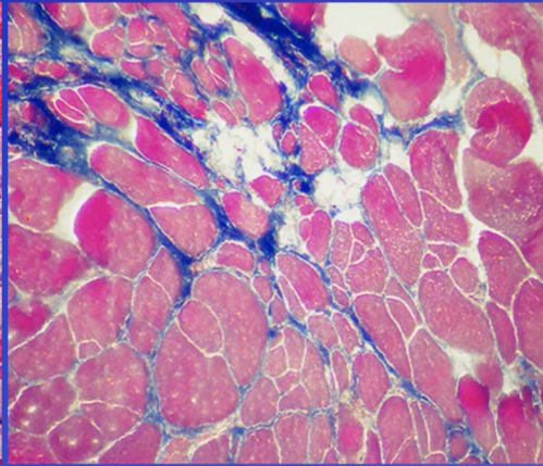
Azan Mallory
