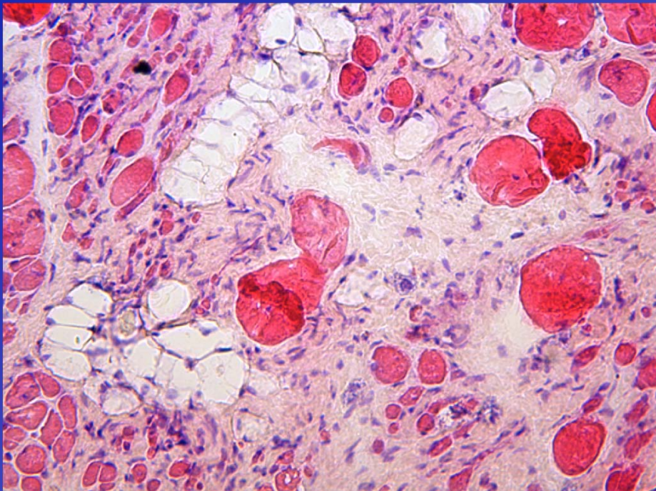
Cont Untreat
