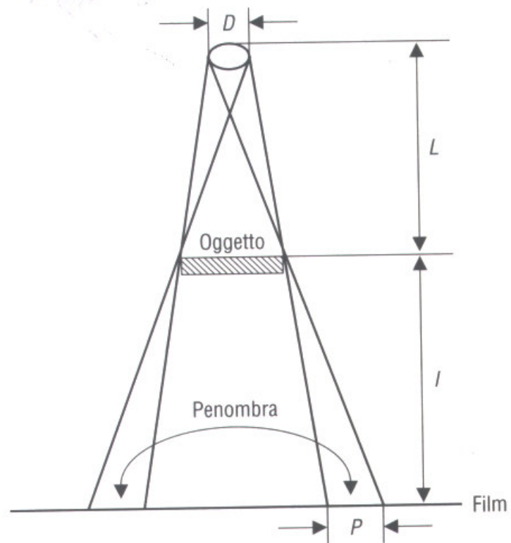
Figura 8.8 Penombra nell'immagine radiografica
