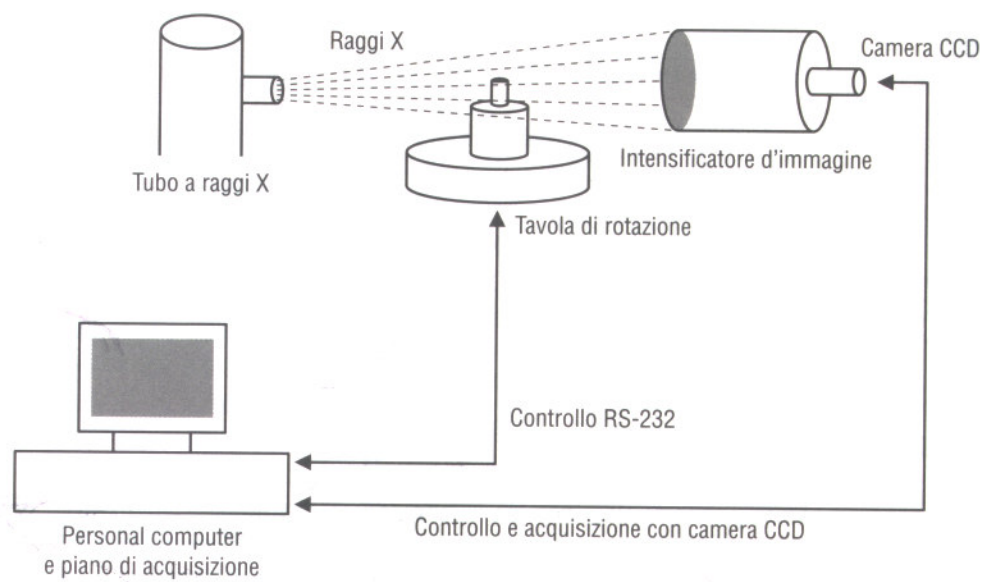
Figura 9.10 Schema di un tomografo computerizzato e fotografia di un tipico tomografo industriale costruito in collaborazione tra l'Istituto di Matematica e Fisica dell'Università di Sassari e la Gilardoni di Mandello al Lario
